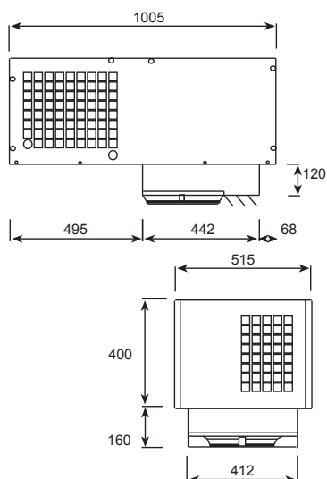
MAATSCHETS 1
