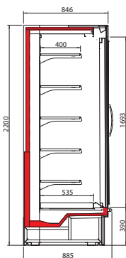
DOORSNEDE BRIONI DOORS H216
