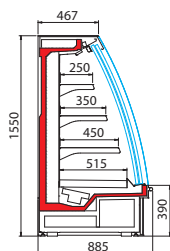
DOORSNEDE PHOENIX2
