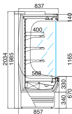
DOORSNEDE TRENT
