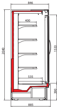
DOORSNEDE BRIONI DOORS
