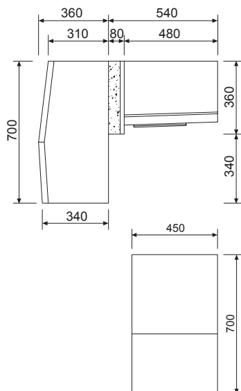
MAATSCHETS 2
