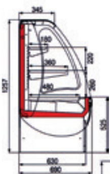
DOORSNEDE H125
