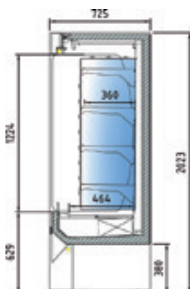
DOORSNEDE CM-6-LE
