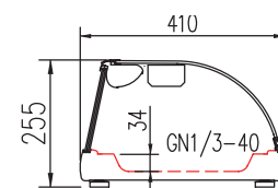
DOORSNEDE BCCS
