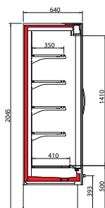
DOORSNEDE DIONE DOORS
