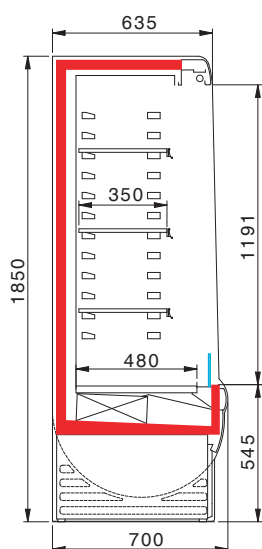
DOORSNEDE VENERE
