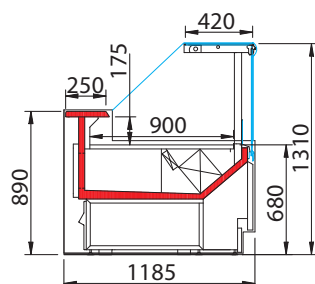
DOORSNEDE MAJOR2 VDA
