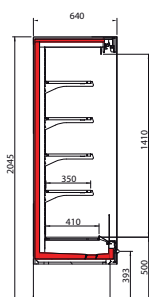
DOORSNEDE DIONE XP EN MP
