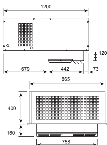
MAATSCHETS 2
