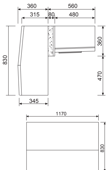
MAATSCHETS 3
