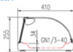
DOORSNEDE BCC
