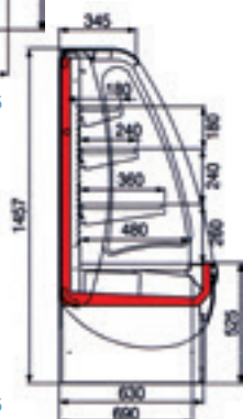
DOORSNEDE H125
