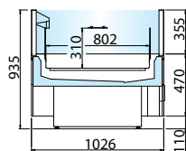
LAVAL G3 BT/TN
