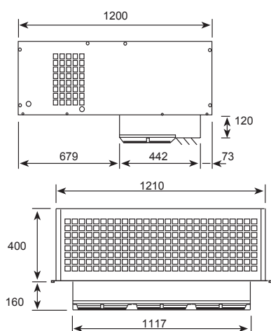
MAATSCHETS 3
