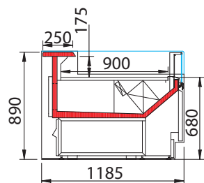
DOORSNEDE MAJOR2 SELF
